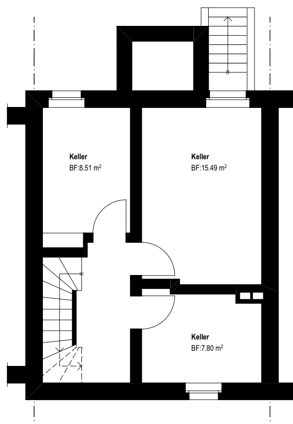
Grundriss Keller
