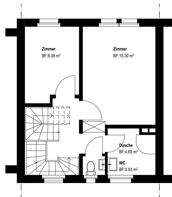
Grundriss 2. Obergeschoss
