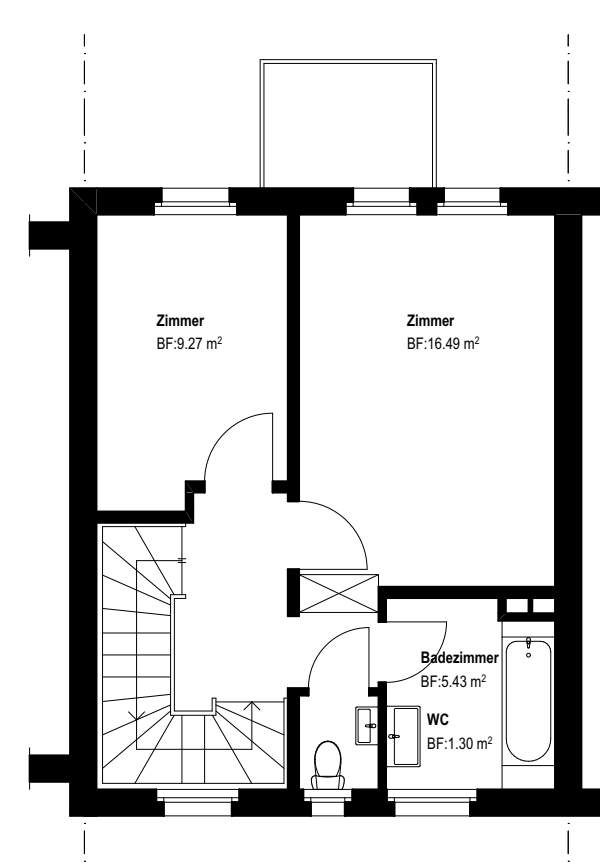
Grundriss 1. Obergeschoss
