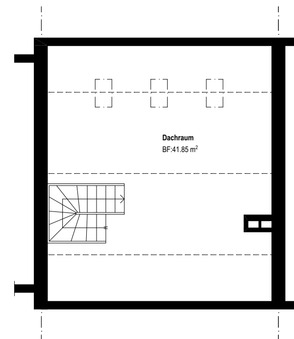
Grundriss Dachgeschoss
